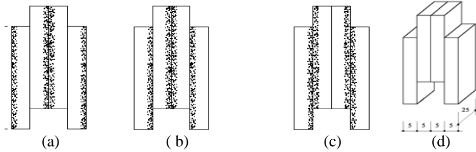
Figura 1: Combinação dos CPs: (a) MM; (b) MC; (c) CC e (d) Esquema do conjunto.
