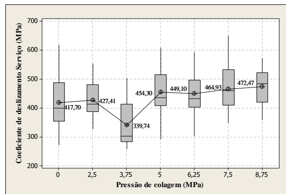
Figura 7: Módulo de deslizamento serviço em função da pressão de colagem.
