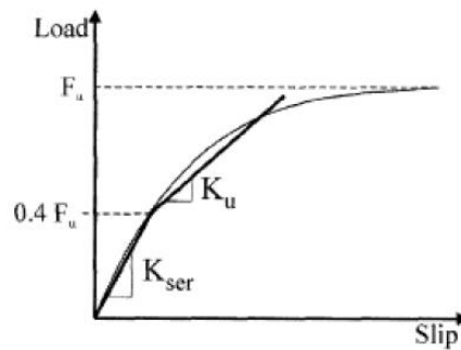
Figura 5: Módulo de deslizamento. Fonte: [10].
