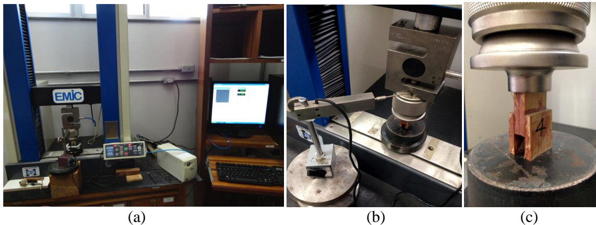
Figura 4: (a) Sistema conectado ao SAD; (b); Medidor de deslocamento e (c) Detalhe do CP e Rótula Universal.
