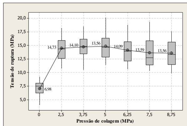
Figura 6: Relação da pressão de colagem com a tensão de ruptura
