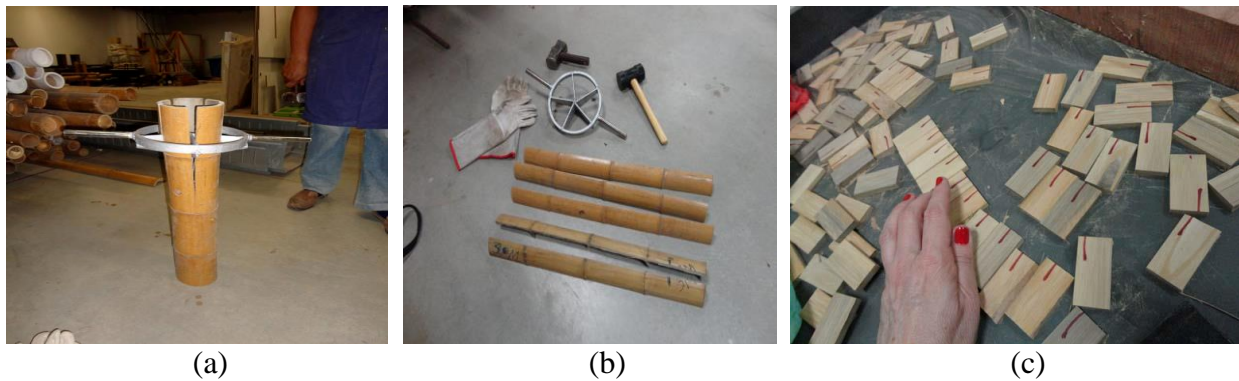
Figura 2: (a) Desdobramento do colmo; (b) Tiras e (c) Lâminas de bambu.
