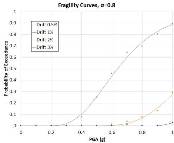
Figura 4: Curvas de Fragilidad para M_w \leq 5.5
