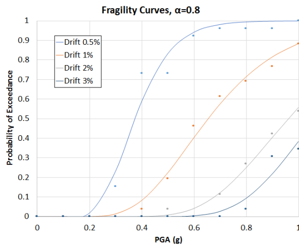
Figura 2: Curvas de Fragilidad para M_w \geq 7.5
