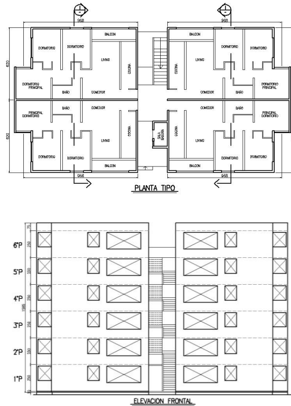
Figura 6: Planta y Elevación de Vivienda Social Típica en Chile
