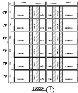
Figura 7: Corte de Vivienda Social Típica en Chile
