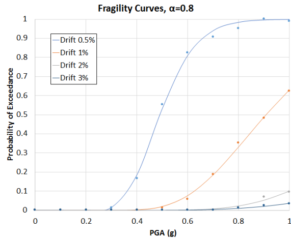
Figura 3: Curvas de Fragilidad para 5.5 \leq M_w \leq 7.5
