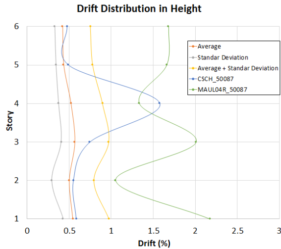
Figura 5: Distribución del Drift Máximo
